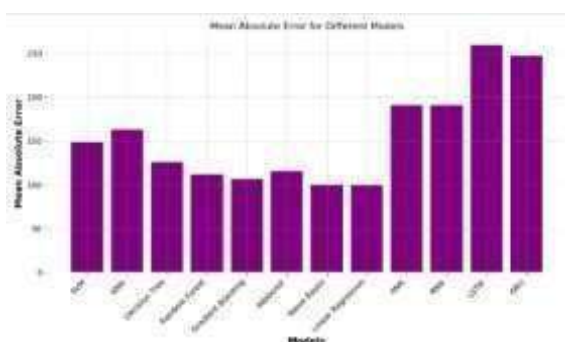
Fig 4: MAE
