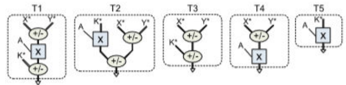
Fig. 3. FCU template library
