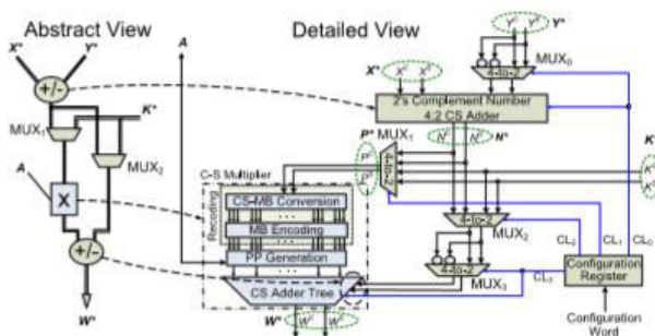
Fig. 2. FCU.
