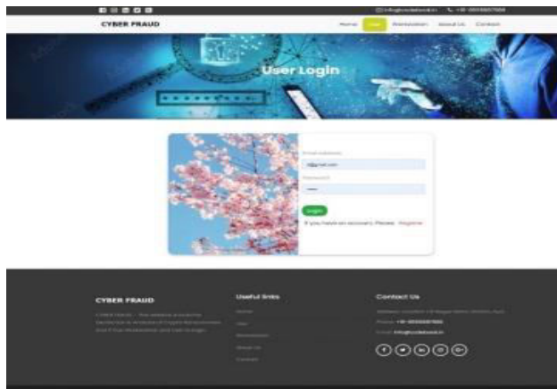
Fig 1:User Login
